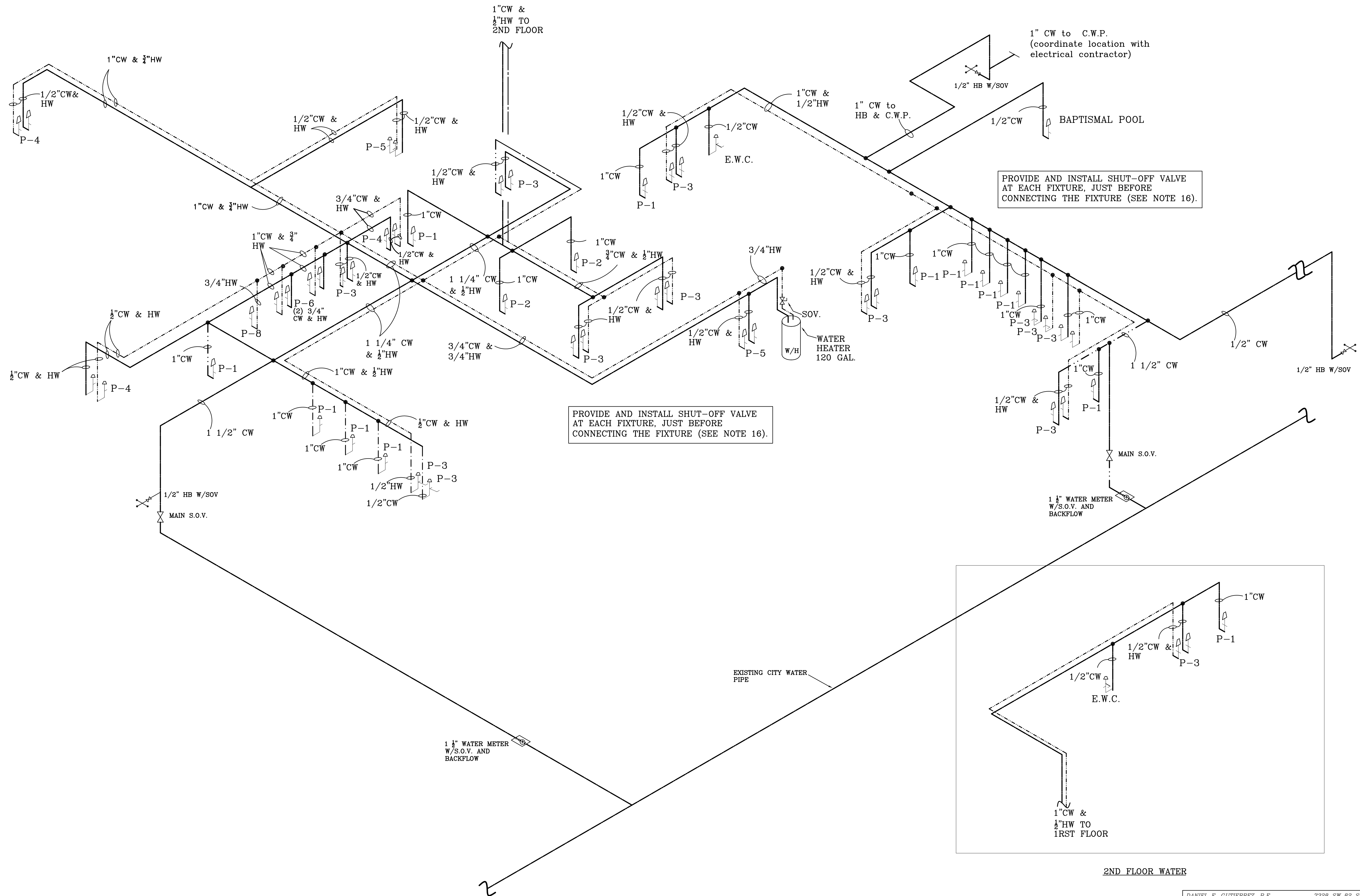
WATER ISOMETRICS SCALE: N.T.S.
